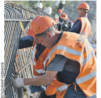
7 августа 2015 года. Реконструкция Звенигородского путепровода
